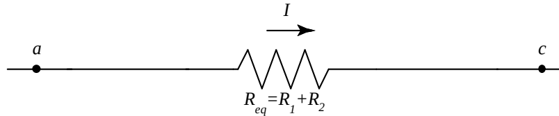
Figura 6.6: As resistências da figura 6.5 podem ser substituídas por uma resistência equivalente R_{eq} = R_1 + R_2 que obtemos a mesma queda de potencial quando a R_{eq} é atravessada pela mesma corrente que no circuito da figura 6.5.
