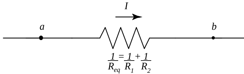
Figura 6.8: As duas resistências da Fig.5. podem ser substituídas por uma resistência equivalente R_{eq} que está relacionada com R_1 e R_2 pela fórmula \frac{1}{R_{eq}} = \frac{1}{R_1} + \frac{1}{R_2} .
