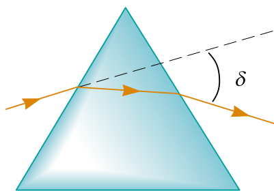
Figura 5.5: Um prisma refracta um raio de luz com um comprimento de onda único por um ângulo \delta .
