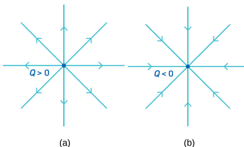
Figura 6.1: Linhas de campo eléctrico em torno de uma carga (a) positiva, (b) negativa.
