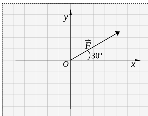
Figura 1.1: Representação gráfica do vector \mathbf{F} .
