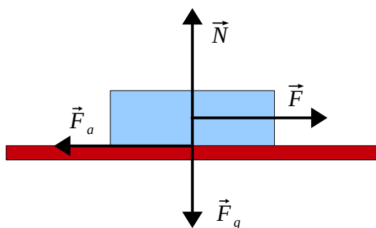
Figura 2.1: Um corpo sujeito à força de atrito.
