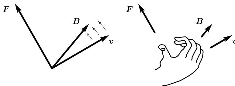
Figura 7.7: A regra da mão direita.
