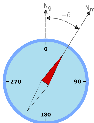
Figura 7.4: A declinação magnética.
