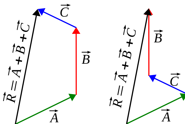
Figura 1.3: Método do polígono.
