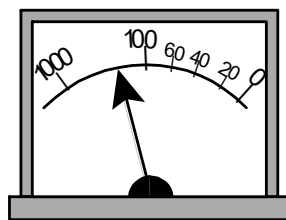
Figura 6.16: Quando uma resistência R é ligada em a e b , a agulha do galvanómetro deflecte uma quantidade que depende do valor de R . A escala do galvanómetro é calibrada de maneira a dar uma leitura em ohms.
