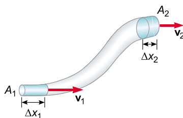
Figura 3.2: Um fluido a mover-se através de um tubo com área de secção recta variável.
