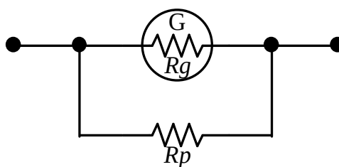
Figura 6.13: Um amperímetro consiste num galvanómetro cuja resistência é R_g e uma pequena resistência em paralelo R_p .
