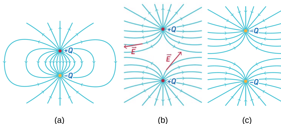
Figura 6.2: Linhas de campo eléctrico para cargas (a) simétricas, (b) iguais positivas, (c) iguais negativas.
