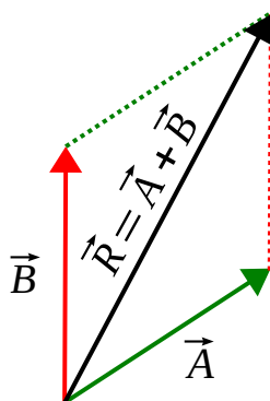
Figura 1.2: Método do paralelogramo.
