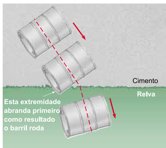
Figura 5.4: Um barril rolando por cima de dois pavimentos diferentes.
