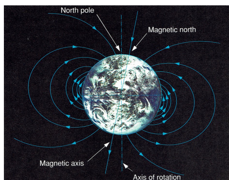
Figura 7.3: O campo magnético terrestre.
