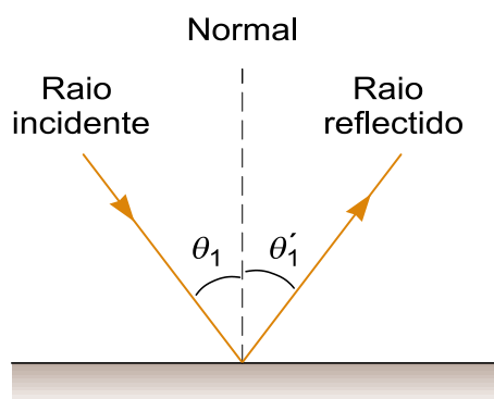
Figura 5.1: O raio incidente, a normal e o raio refletido estão todos no mesmo plano.
