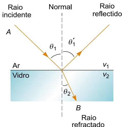
Figura 5.2: O raio incidente, a normal, o raio reflectido e o raio refractado estão todos no mesmo plano.
