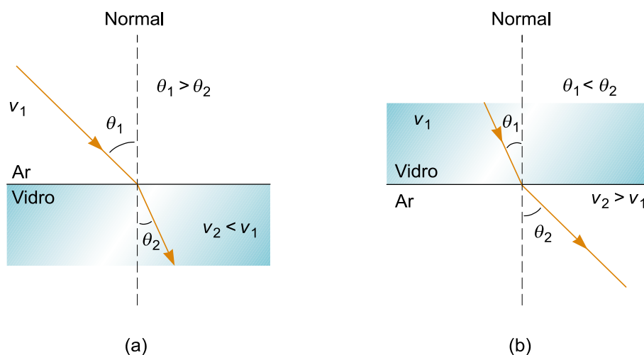
Figura 5.3: (a) Luz move-se de um material em que a sua a velocidade é elevada para um material em que a sua velocidade é inferior, o raio inclina-se de forma a aproximar-se da normal. (b) Luz move-se a partir de um material no qual a sua velocidade é lenta para um material em que se move mais rapidamente, o raio inclina-se de forma a afastar-se da normal.
