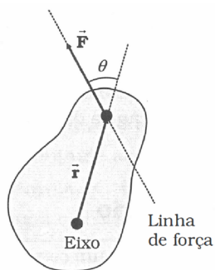
Figura 2.2: Momento de uma força.
