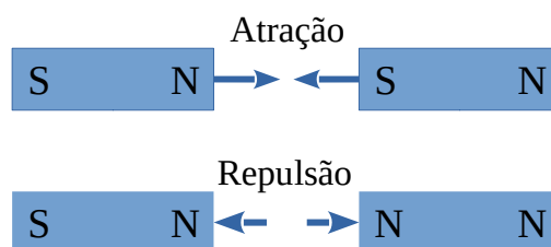
Figura 7.5: A atração e repulsão entre ímãs.
