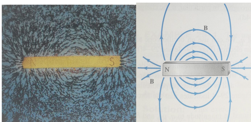
Figura 7.6: Campo magnético B perto de um íman e as linhas de indução magnética. À esquerda o que acontece na realidade, à direita o que preconiza a teoria.
