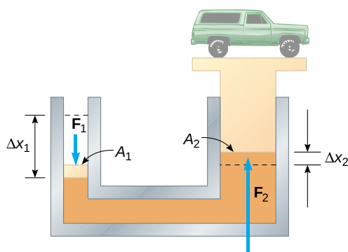
Figura 3.1: Diagrama de uma prensa hidráulica.
