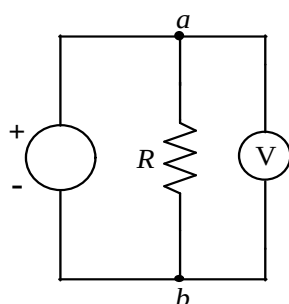
Figura 6.12: Para medir a queda de potencial numa resistência, um voltmímetro é colocado em paralelo com a resistência para que a queda de potencial seja a mesma no voltmímetro e na resistência.
