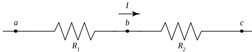
Figura 6.5: Duas resistências em série são atravessadas pela mesma corrente.
