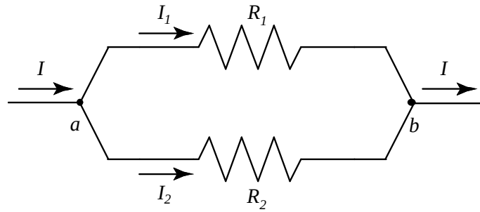
Figura 6.7: Duas resistências estão em paralelo quando estão juntamente ligadas em ambas as extremidades de maneira que a queda de potencial é a mesma nas duas.
