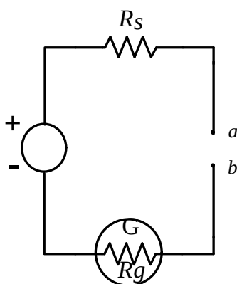
Figura 6.15: Um ohmímetro consiste numa bateria em série com um galvanómetro e uma resistência R_s , escolhida de modo a que quando os terminais a e b são postos em curto-circuito, a corrente através do galvanómetro provoca uma deflexão completa na escala escolhida.
